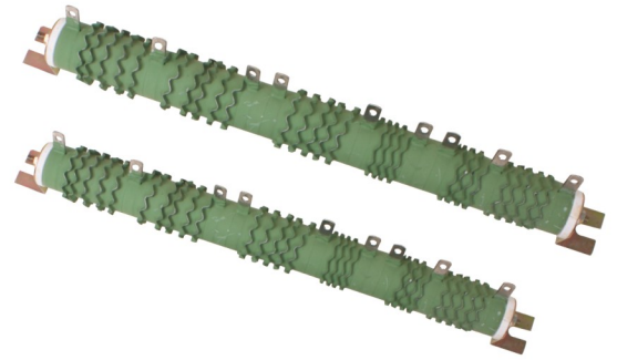
波浪型 RIBBON WIREWOUND RESISTOR
