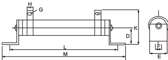
平面繞線型 PLATE RESISTOR
